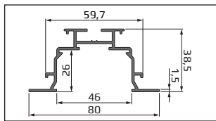
Anbringung mit Sonderzubehör Einbauprofil. (Schienenbefestigung mit Kunststoffclip.)
