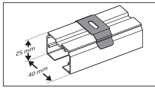
Anbringung mit Deckenhalter.
